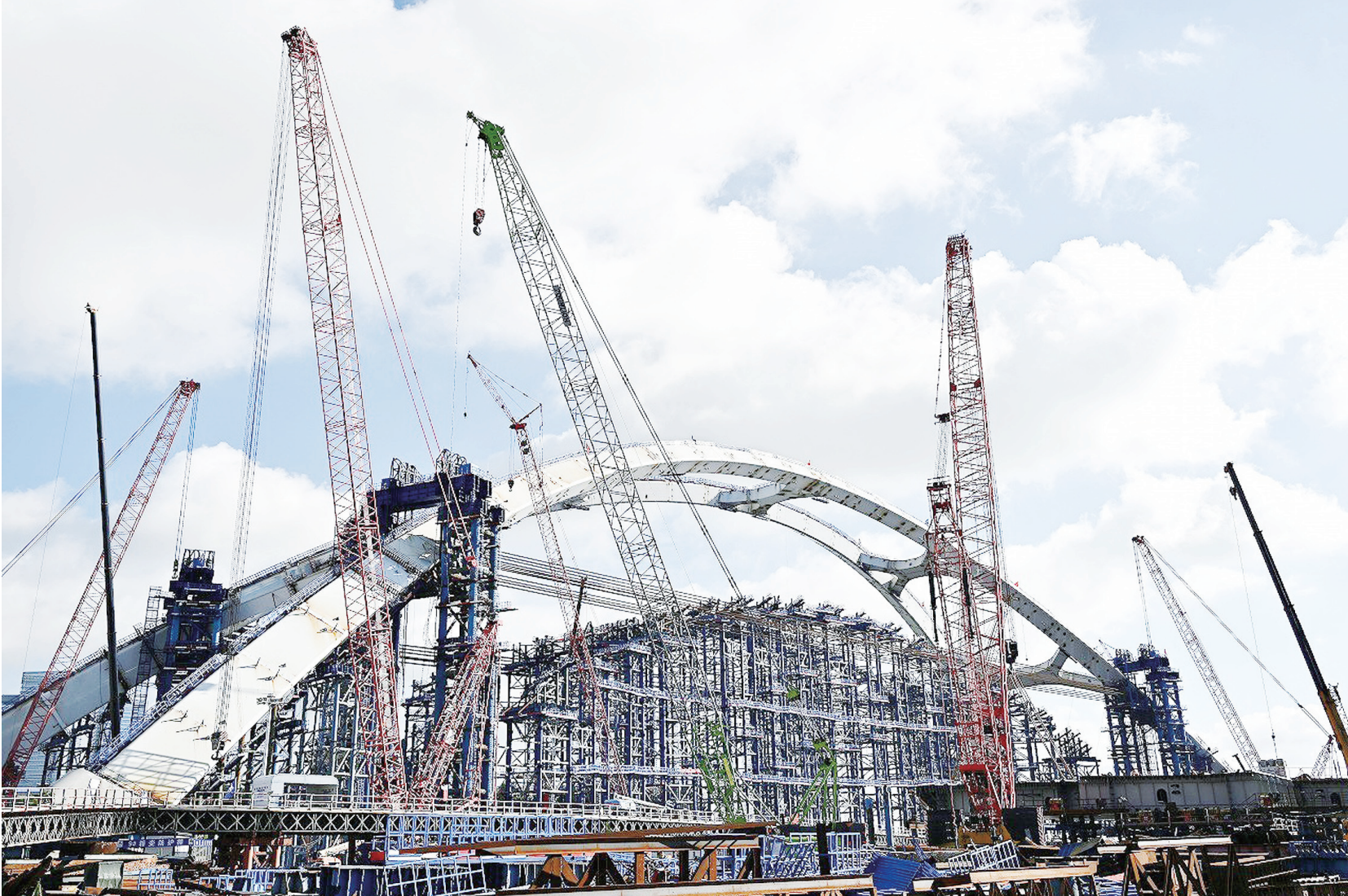
10400噸創世界紀錄 廈金大橋（廈門段）觀音山互通主線橋拱肋合龍 7月8日，廈金大橋（廈門段）建設再迎關鍵性節點——觀音山互通主線橋重達10400噸的中段拱肋，完成30米整體精準提升，順利與邊段拱肋對接合龍。觀音山互通主線橋是廈金大橋（廈門段）關鍵控制性工程之一，項目採用魚骨梁挑起外側匝道橋設計方案，規避在沙灘設墩。據介紹，此次合龍的中段拱肋提升總重量達10400噸，創下同類橋樑鋼拱肋整體提升重量最大的世界紀錄。圖為觀音山互通主線橋拱肋合龍後的場景。 <中新社>
